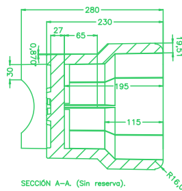
SECCIÓN A-A. (Sin reserva).
