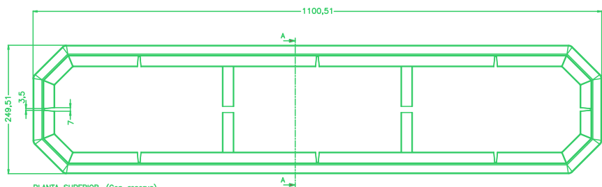
PLANTA SUPERIOR. (Con reserva)
