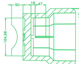
SECCIÓN A-A. (Con reserva).
