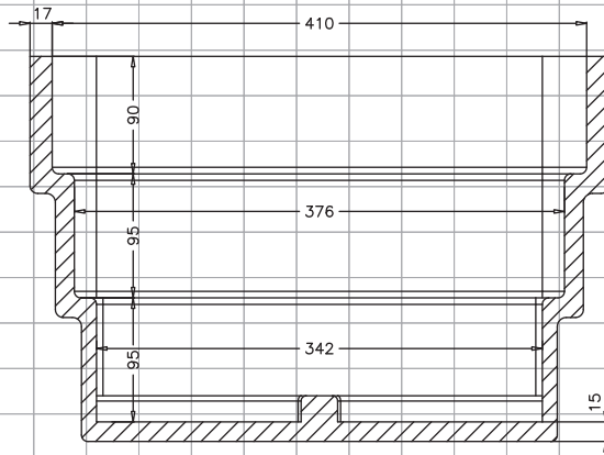
SECCIÓN A-A
