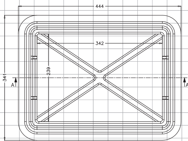
PLANTA SUPERIOR.
