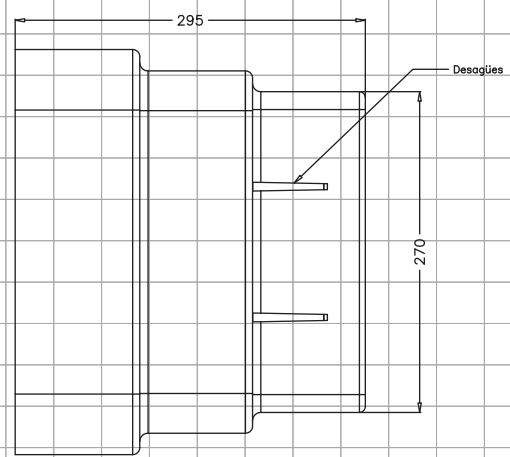
ALZADO LATERAL.
