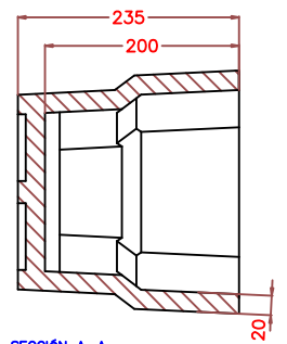
SECCIÓN A-A.
