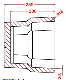
SECCIÓN A-A.
