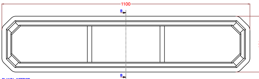
PLANTA INFERIOR.
