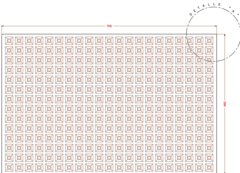
PLANTA SUPERIOR.
