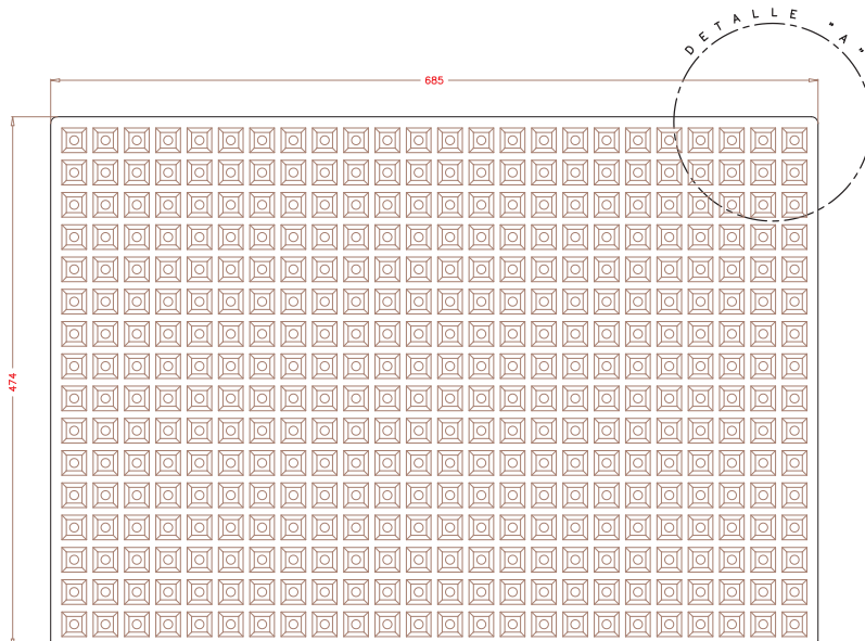
PLANTA SUPERIOR.
