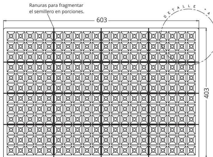
PLANTA SUPERIOR
