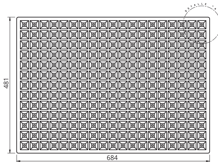
PLANTA SUPERIOR
