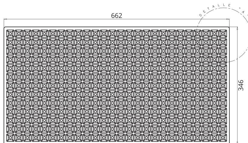
PLANTA SUPERIOR
