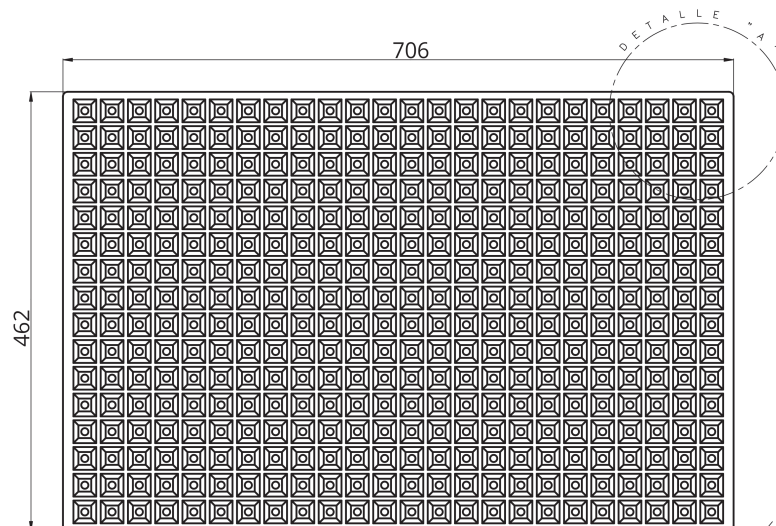
PLANTA SUPERIOR
