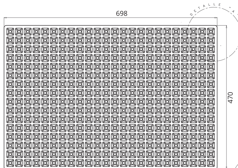
PLANTA SUPERIOR
