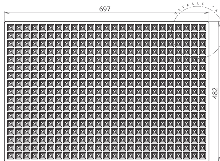
PLANTA SUPERIOR
