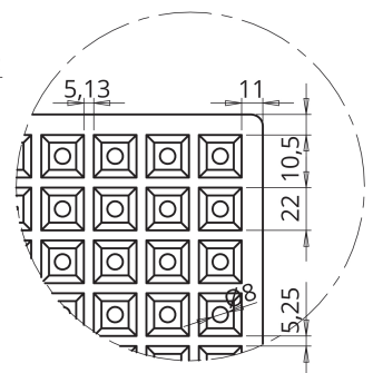
DETALLE A
