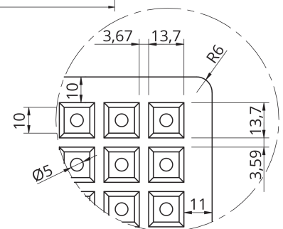
DETALLE A
