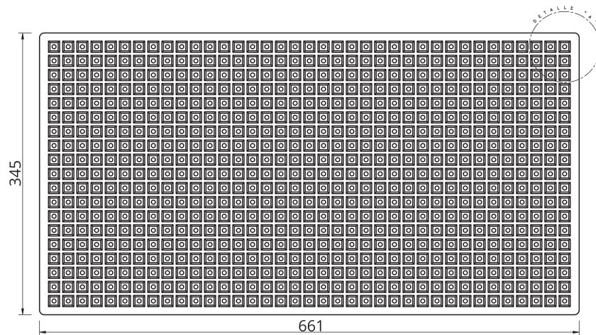
PLANTA SUPERIOR
