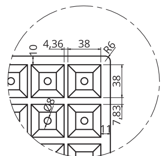
DETALLE A
