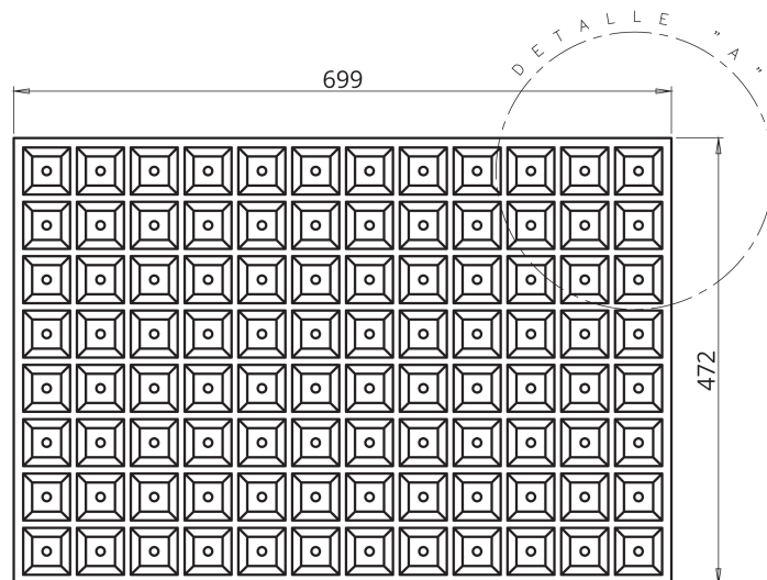
PLANTA SUPERIOR
