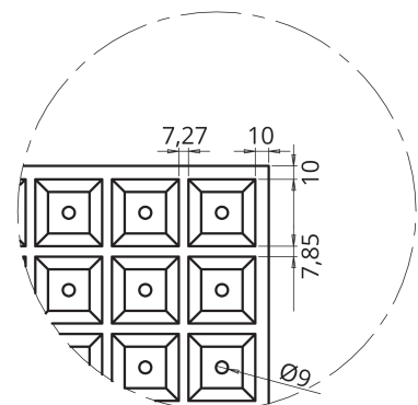
DETALLE A
