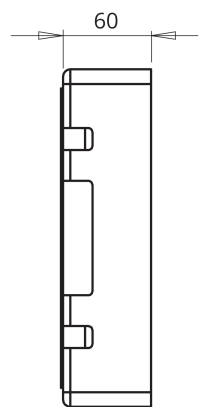
ALZADO LATERAL
