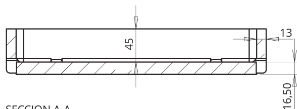
SECCION A-A
