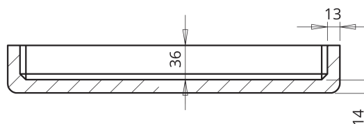
SECCION A-A
