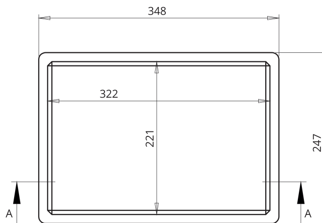
PLANTA SUPERIOR
