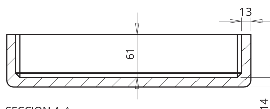
SECCION A-A
