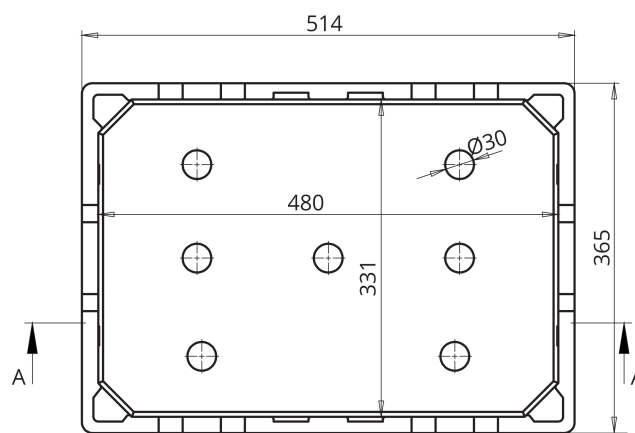
PLANTA SUPERIOR
