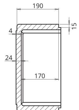
SECCIÓN A-A
