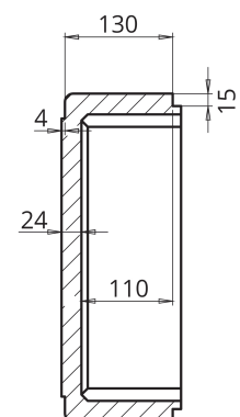
SECCIÓN A-A
