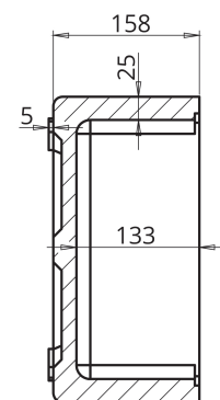
SECCION A-A
