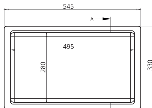
PLANTA SUPERIOR
