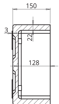
SECCION A-A
