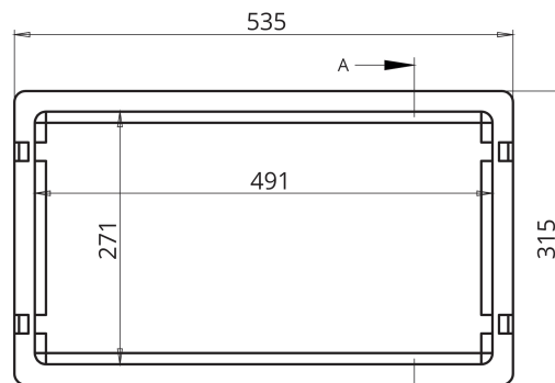
PLANTA SUPERIOR
