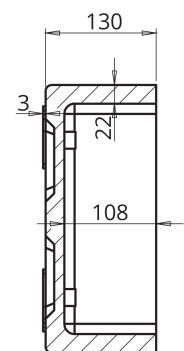
SECCION A-A
