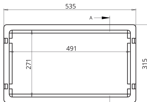
PLANTA SUPERIOR
