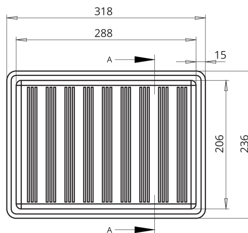
PLANTA SUPERIOR
