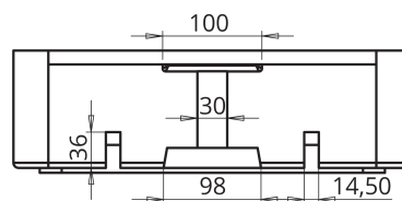
ALZADO FRONTAL
