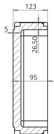
SECCION A-A
