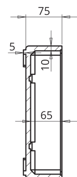
SECCION A-A
