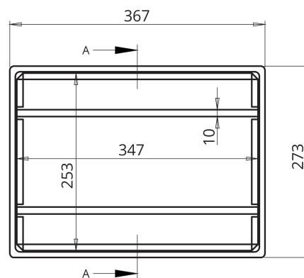
PLANTA SUPERIOR
