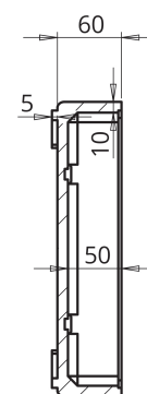
SECCION A-A
