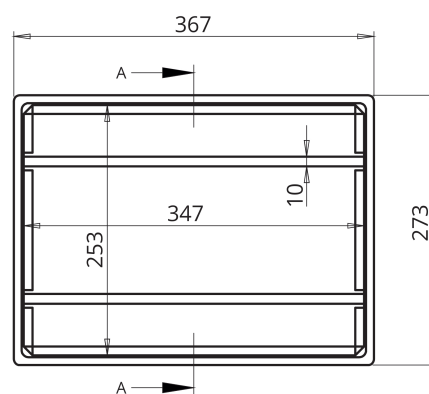
PLANTA SUPERIOR
