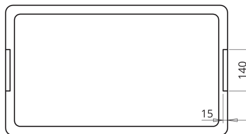
PLANTA INFERIOR
