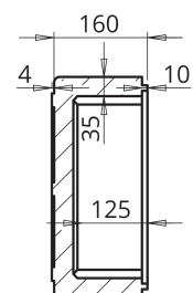
SECCION A-A
