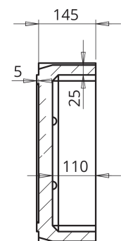
SECCION A-A
