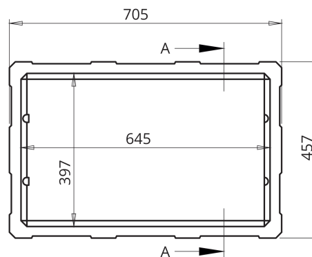
PLANTA SUPERIOR
