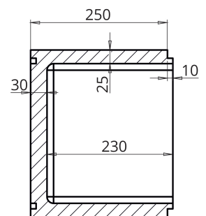
SECCION A-A
